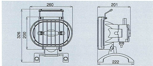
H326×W260×D222mm ML-105K (5m電線仕様) ● コンパクトな床置きタイプ ● 持ち運びに便利な持ち手付
