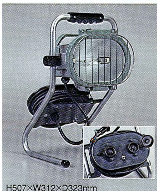
H507×W312×D323mm MLD-107K (7m電線仕様) ● 防雨型コードドラム付 ● コンセントは2個まで同時使用可 ● 上下首振り可能
