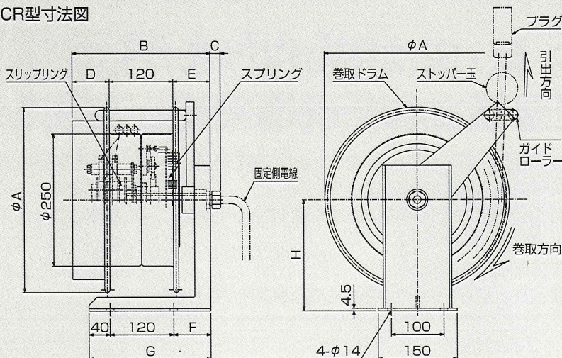
FCR型寸法図
