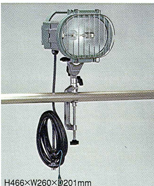
H466×W260×D201mm MLV-105K (5m電線仕様) ● バースでしっかり固定 ● 有効締付幅100mm
