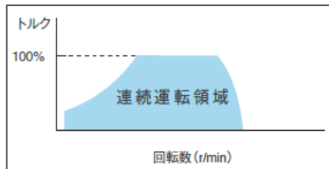
■単相可変速モータ
